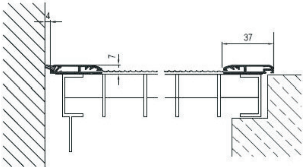
Schnitt bei Montage mit seitlicher Bürste
