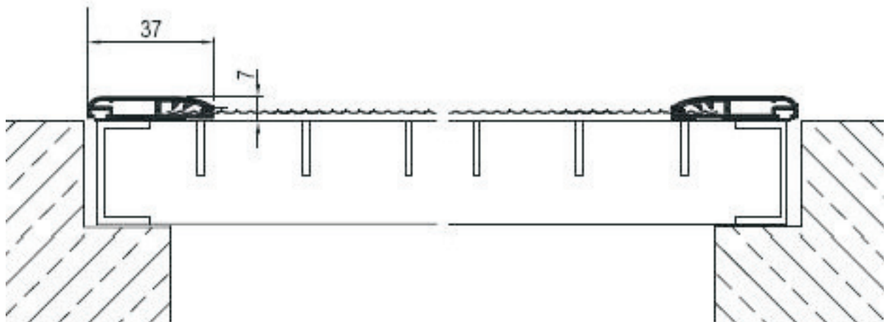
Schnitt bei Montage ohne seitliche Bürste
